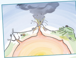
40 Vulkanausbruch
